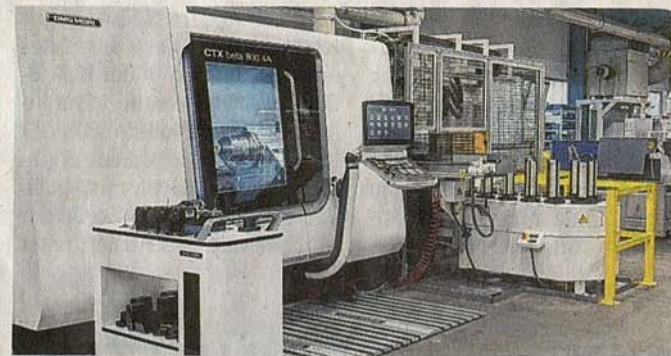
Vollautomatisierte Fertigungstechnik CTX beta 800 4A
